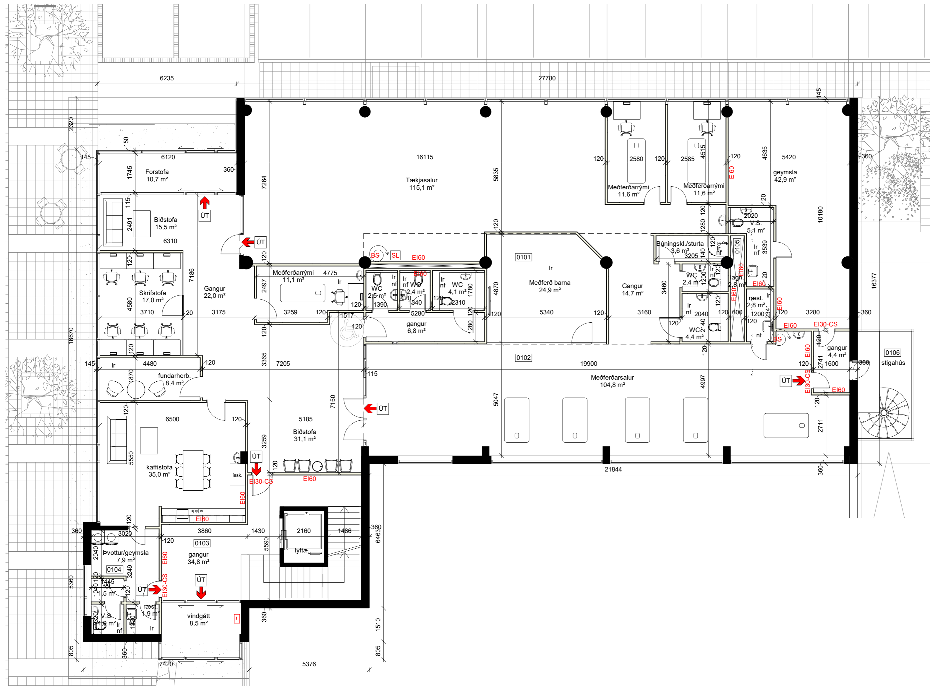
grunnmynd 1. hæðar 1 : 100
